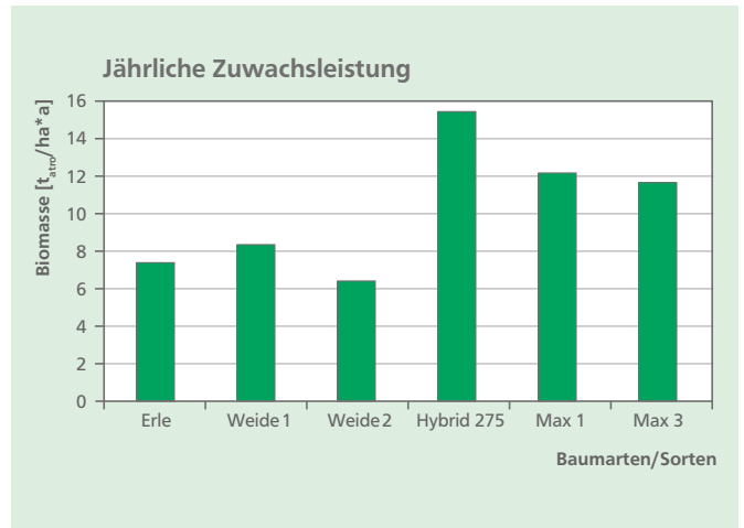
Beispiel: Massenleistung der Versuchsfläche Coburg im 3. Umtrieb
