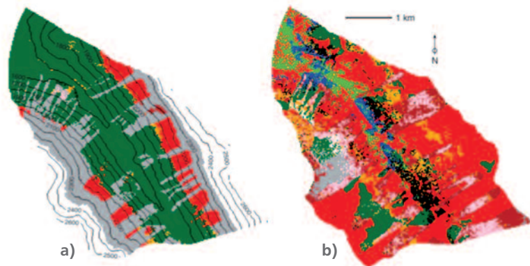
Abbildung 4: Verteilung dominanter Baumarten im Dischmatal (Schweiz), simuliert mit LandClim für (a) aktuelles Klima (3,2 °C Jahresmitteltemperatur, 900 mm Jahresniederschlag) und (b) ein Klimaszenario (6,2 °C Jahresmitteltemperatur, 700 mm Jahresniederschlag (aus: Pretzsch, Grote, Reineking, Rötzer, Seifert (2008): Models for Forest Ecosystem Management: A European Perspective. Annals of Botany 101: 1065–1087)
