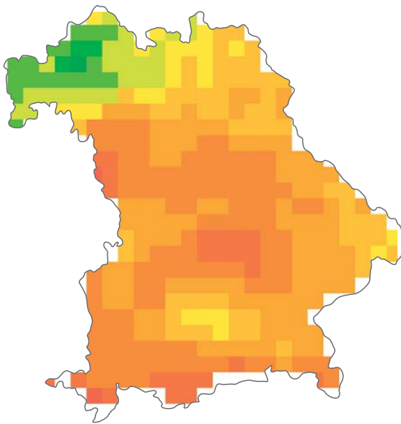
Abbildung 3: Mittlere Änderungen des Jahresniederschlags für das Szenario B1 für die Jahre 2071–2100 gegenüber dem Referenzzeitraum 1961–1990 für WETTREG (links) und REMO (rechts)
