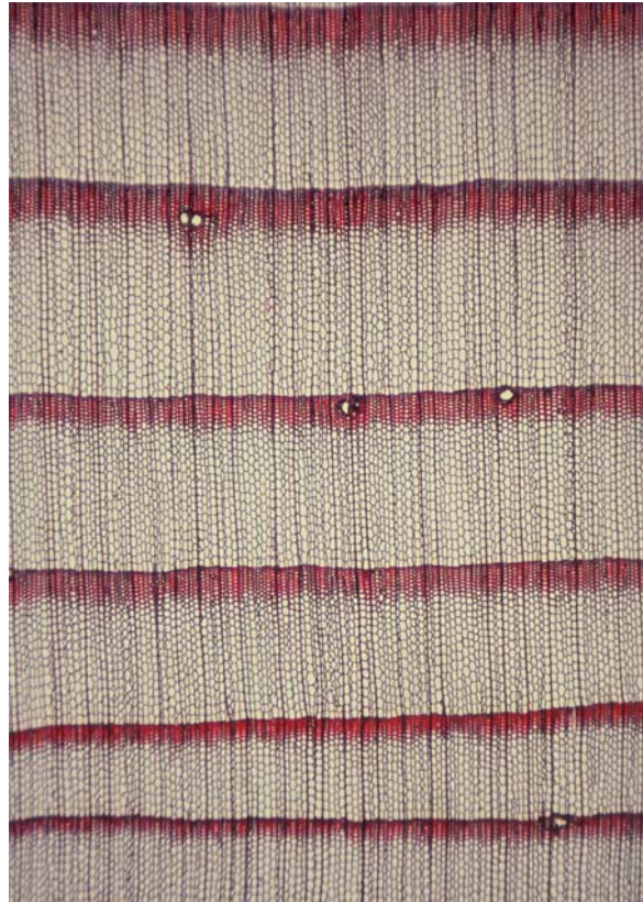
Abbildung 4: Lärche, Querschnitt; Mikrobild im Maßstab 25:1 (Foto: D. Grosser)
